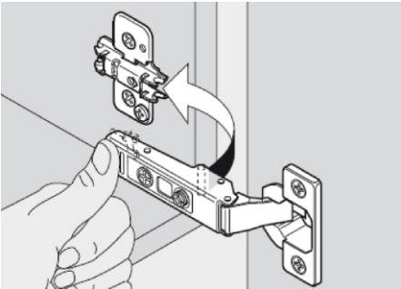
DOOR INSTALL
