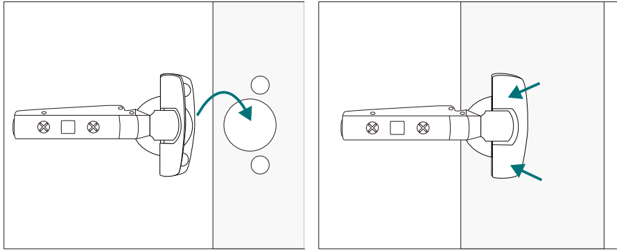
DOOR INSTALL
